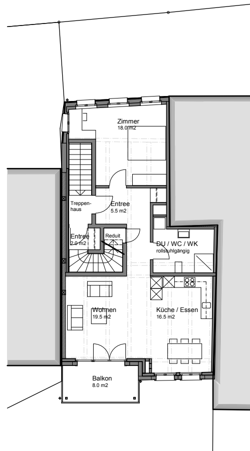
Grundriss Obergeschoss
