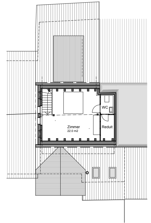
Grundriss 2. Dachgeschoss
