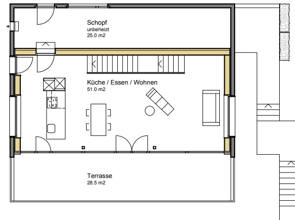
Grundriss Obergeschoss
